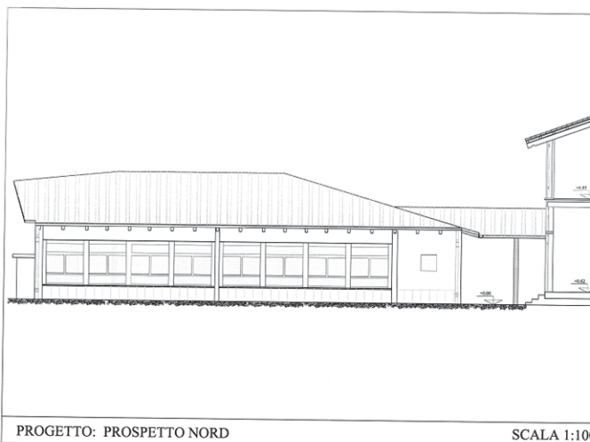
PROGETTO: PROSPETTO NORD SCALA 1:10
